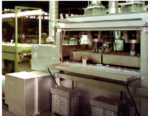
Figura 7: Foto forno de placas de endireitamento [3].
