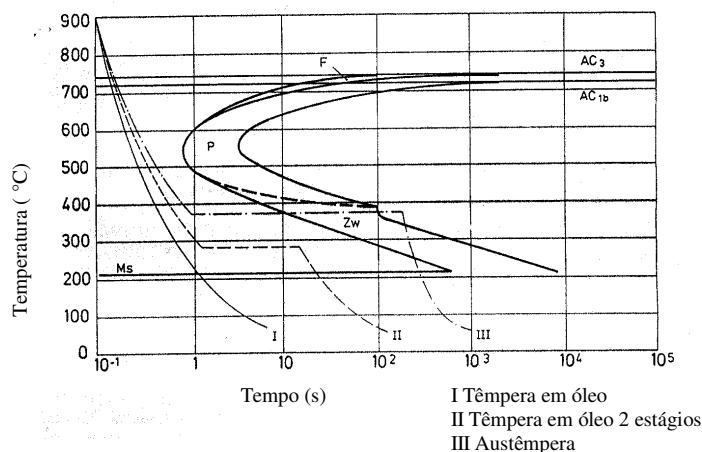
Figura 4: Diagrama T.T.T. de um aço SAE 1075 [5].
