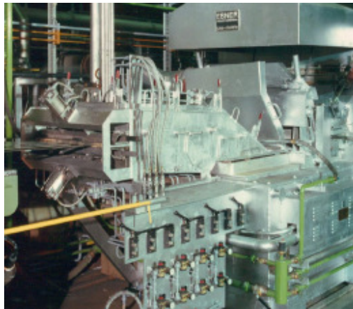
Figura 5: Foto do tanque de resfriamento metálico [3].
