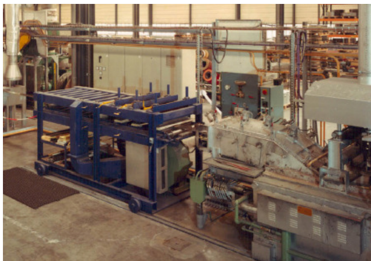
Figura 6: Foto das seções de resfriamento metálico e resfriamento com jatos de ar [3].
