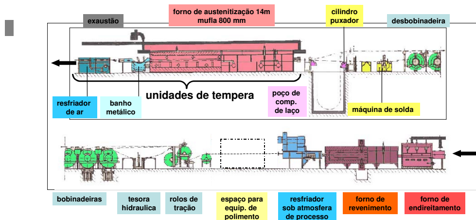
Figura 2: Representação esquemática de uma linha completa de beneficiamento contínuo de tiras [3].
