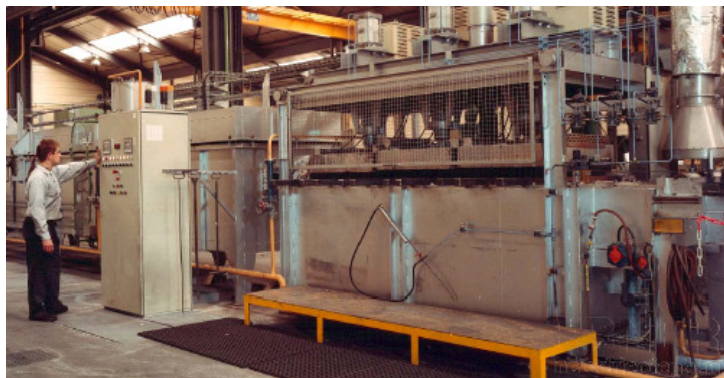
Figura 8: Foto de forno de endireitamento e de revenimento [3].
